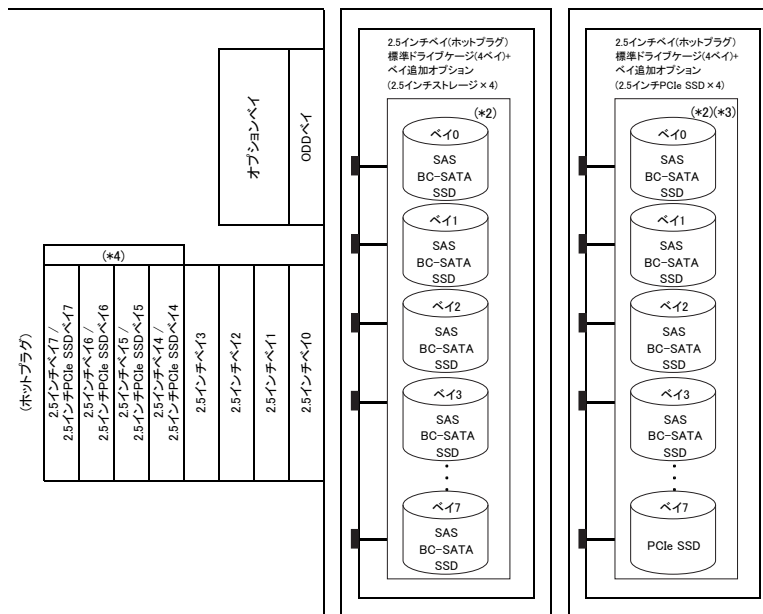
【サーバ前面】→
