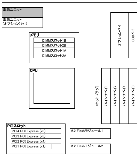
【サーバ前面】→
